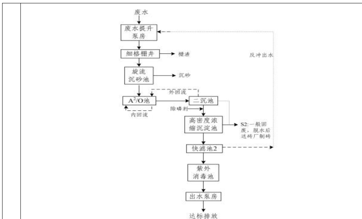
图 4-2 建湖县城东污水厂一期污水处理工艺流程图
