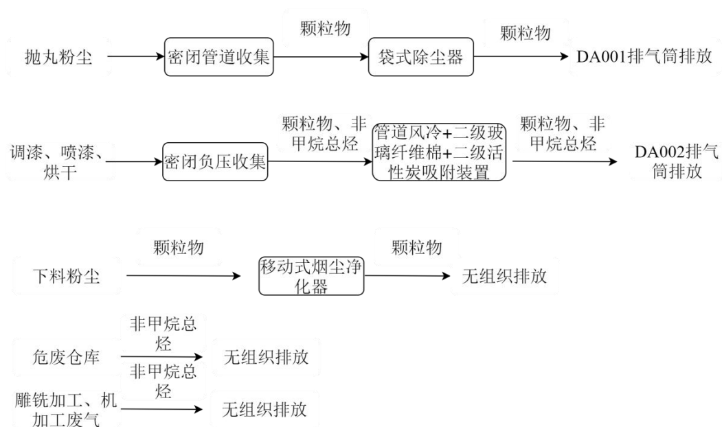
图 4-1 项目废气处理工艺流程
