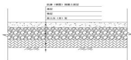
图 4-6 一般防渗区地面防渗结构示意图
