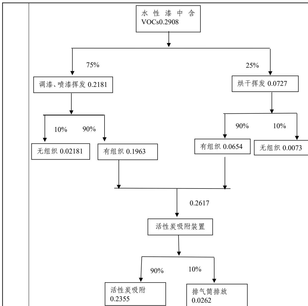
图 2-2 项目 VOCs 物料平衡图 (t/a)
