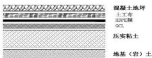
图 4-5HDPE 膜与基础连接示意图
