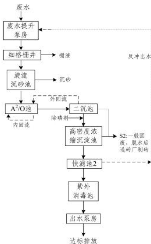
图 4-3 建湖县城东污水处理厂工艺流程图
