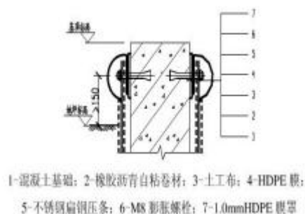
图 4-4 设计 HDPE 膜单层防渗结构示意图
