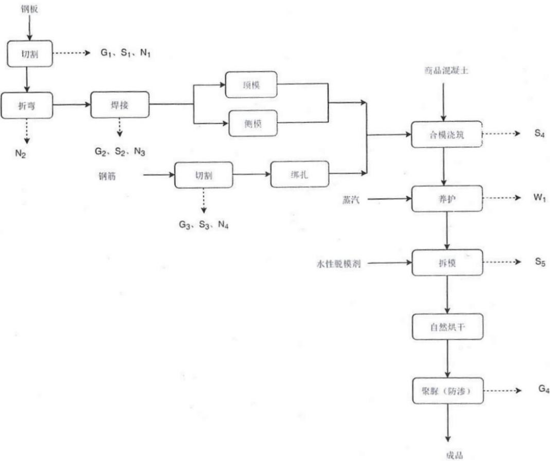
图 2-3 现有项目生产工艺流程及产污环节示意图
