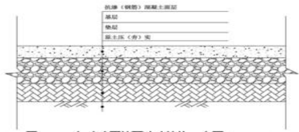
图 4-6 一般防渗区地面防渗结构示意图
