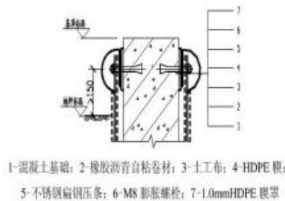
图 4-5 HDPE 膜与基础连接示意图
