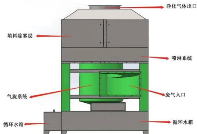
图 4-2 气旋喷淋塔结构简图
