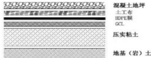
图 4-4 设计 HDPE 膜单层防渗结构示意图
